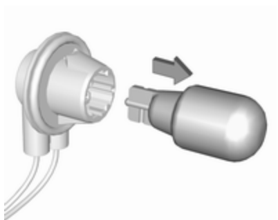
Rückfahrleuchte
