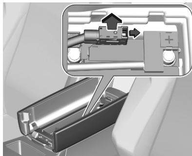
7. PHEV : débloquer et déposer le connecteur de la borne négative.
