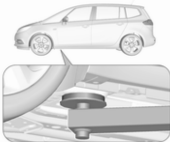
Position du bras arrière du pont élévateur centrée sous le creux du seuil.
