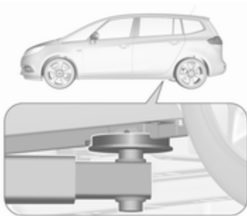
Position du bras arrière du pont élévateur centrée sous le creux du seuil.
