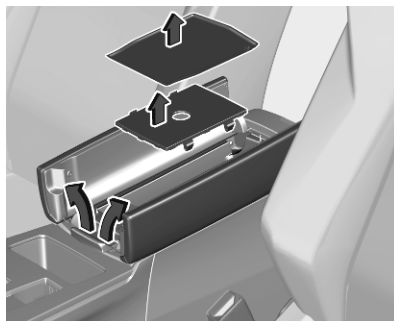
6. Hibridno vozilo: Odstranite dno.
