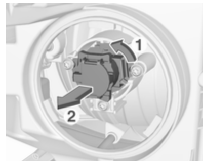
1. Zasukajte pokrov v levo in ga odstranite.
