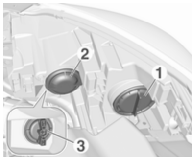
Kratka luč (1), zunanja žarnica. Dolga luč (2), notranja žarnica. Prednji smernik (3)
