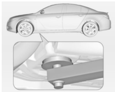
下車體升降台的前臂位置。
