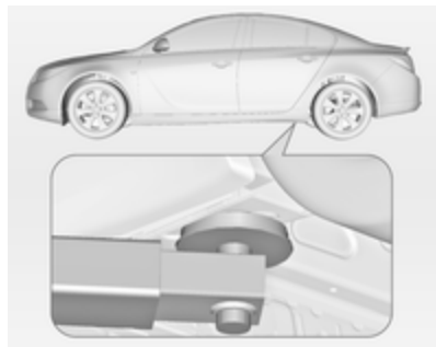
下車體升降台的後臂位置。
